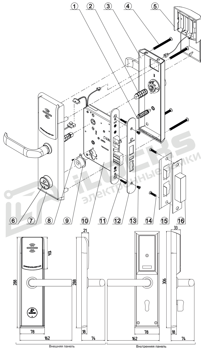
Рисунок №1 – Структурная схема (спецификация) и габариты замков типа iLOCKS IS8005AB3
