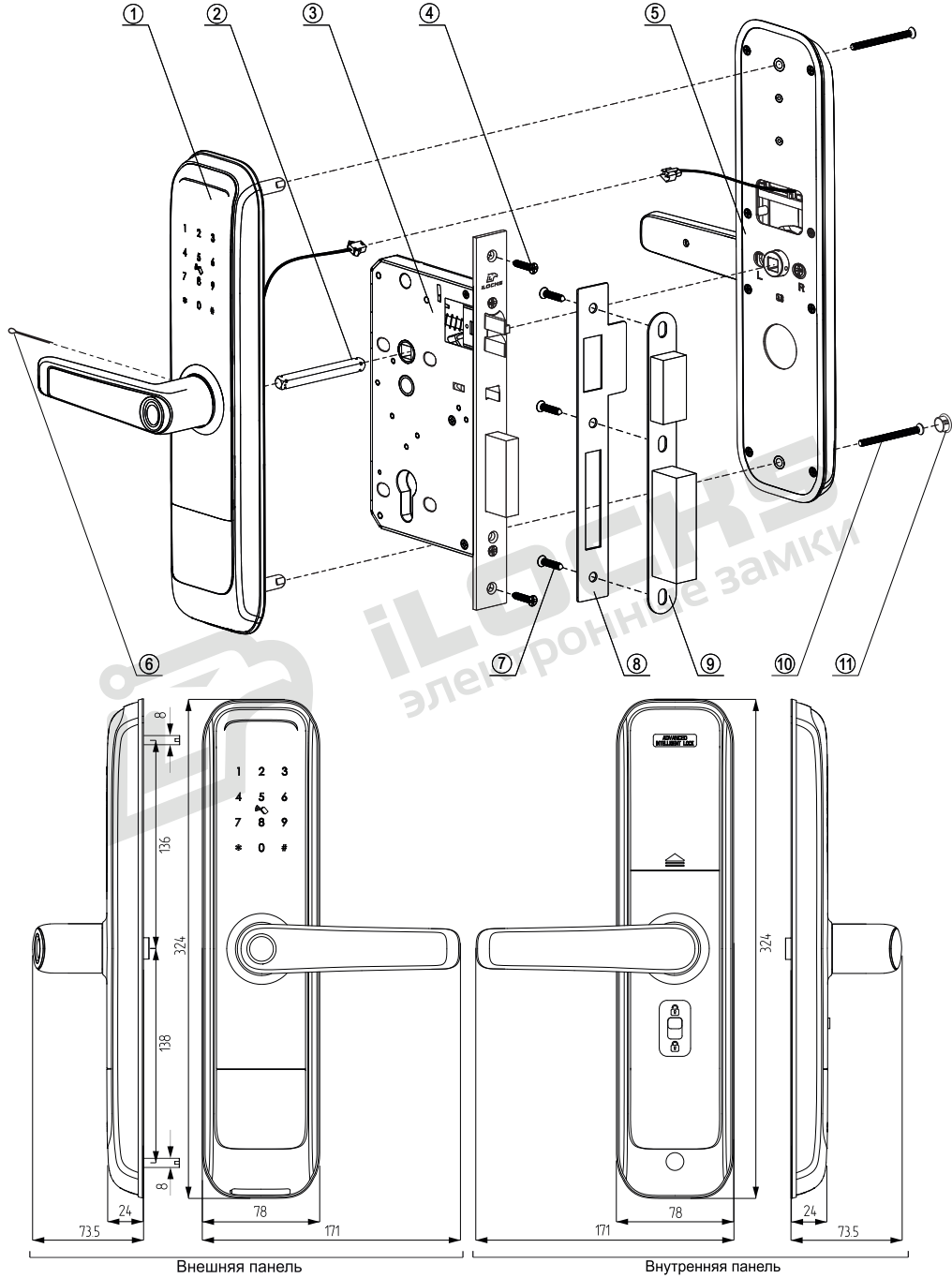
Рисунок №1 – Структурная схема (спецификация) и габаритные характеристики замков типа IS240F 433+BLE
