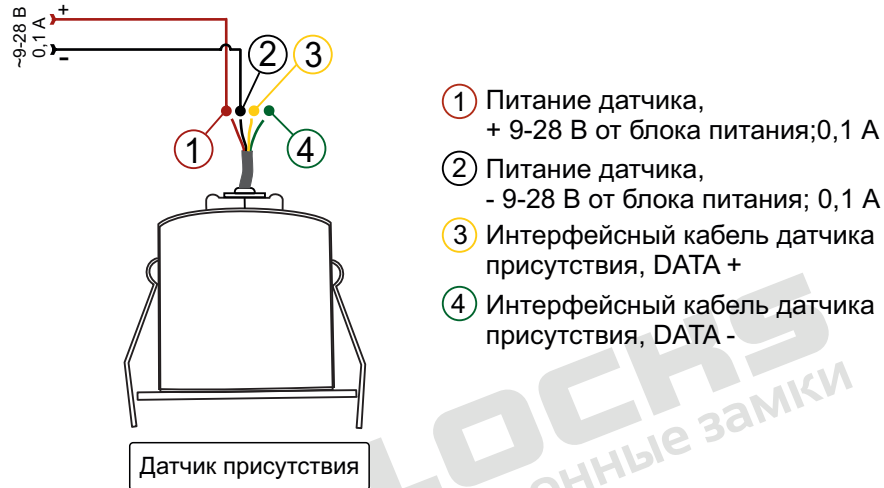
Рисунок №1. Контакты датчика присутствия
