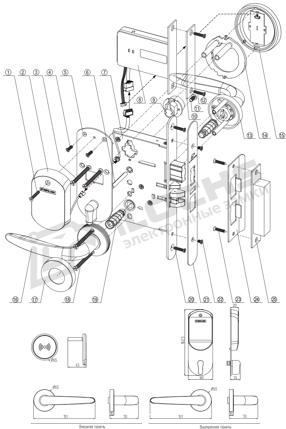
Рисунок №1 – Структурная схема (спецификация) замков типа iLOCKS IS180
