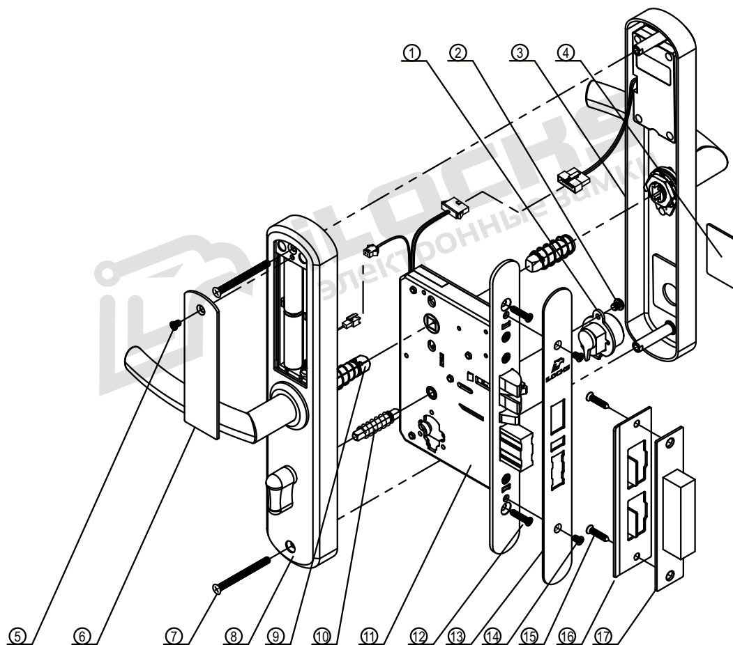
Рисунок №1 – Структурная схема (спецификация) замков типа iLOCKS IS200
